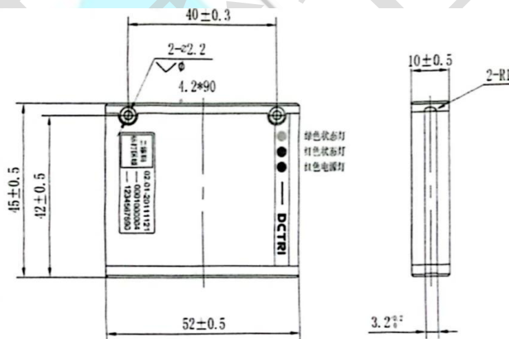
图 2-3 SAM 模块尺寸图
